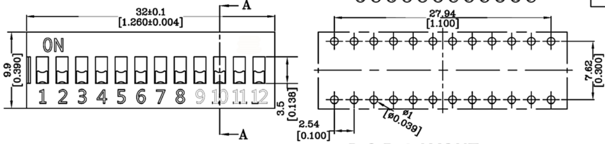
P.C.B LAYOUT
